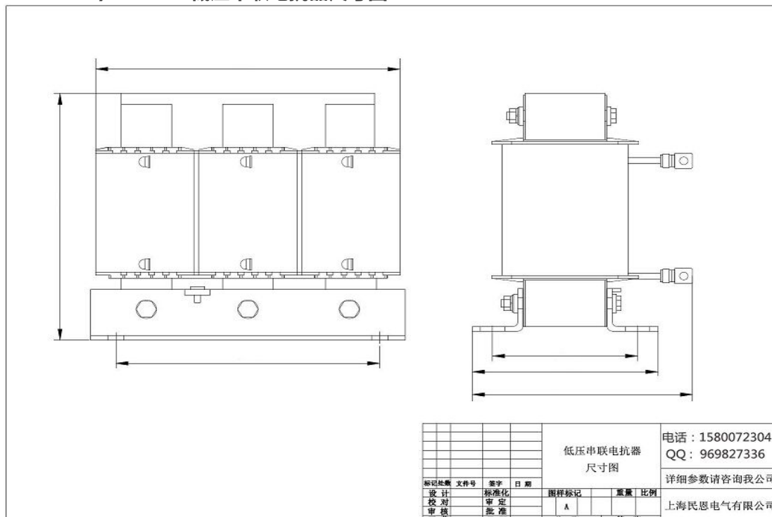
CKSG-2.1/0.48-7%低压串联电抗器尺寸图：
