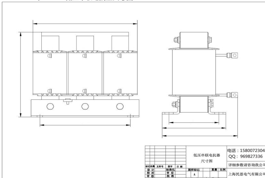
CKSG-1.75/0.4-7%低压串联电抗器尺寸图：
