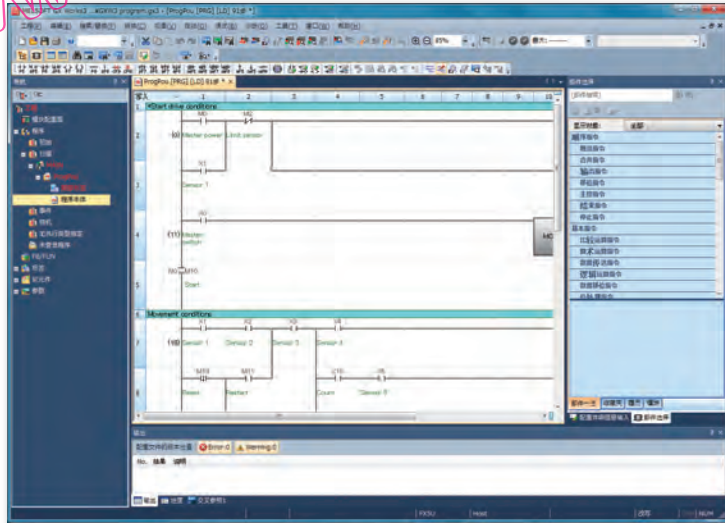
梯形图语言
