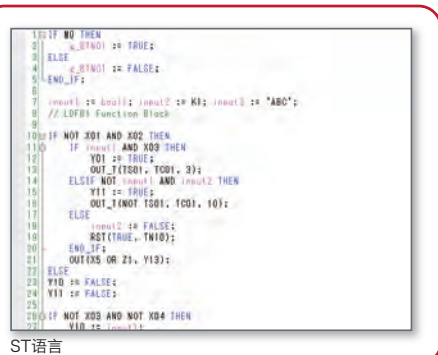
ST语言
