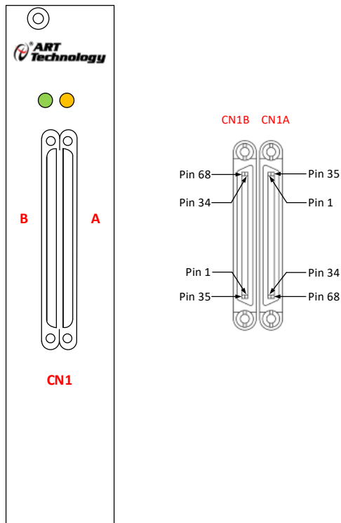
图 3-3-2 PXIe 连接器接口示意图
