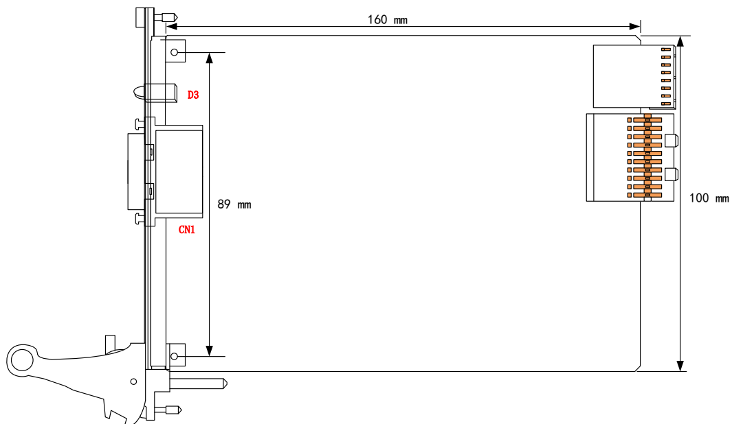
图 3-2-1 板卡尺寸图
