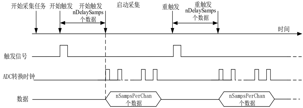
图 8-2-7 重触发
