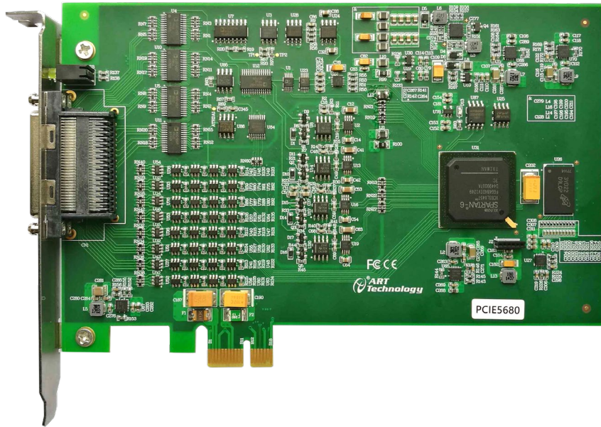
图 3-1-1 PCIe568x 板卡正面图
