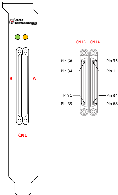
图 3-3-1 PCIe 连接器接口示意图
