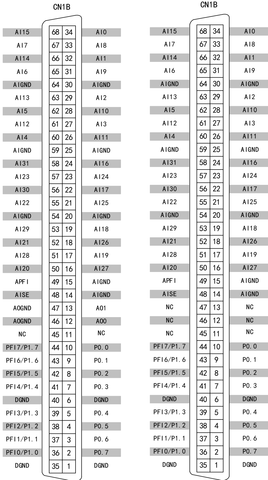
图 3-3-3 连接器引脚定义
