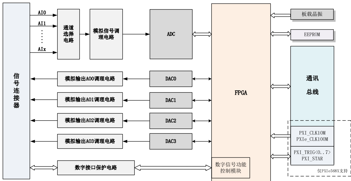
图2-2-1 568X系统框图
